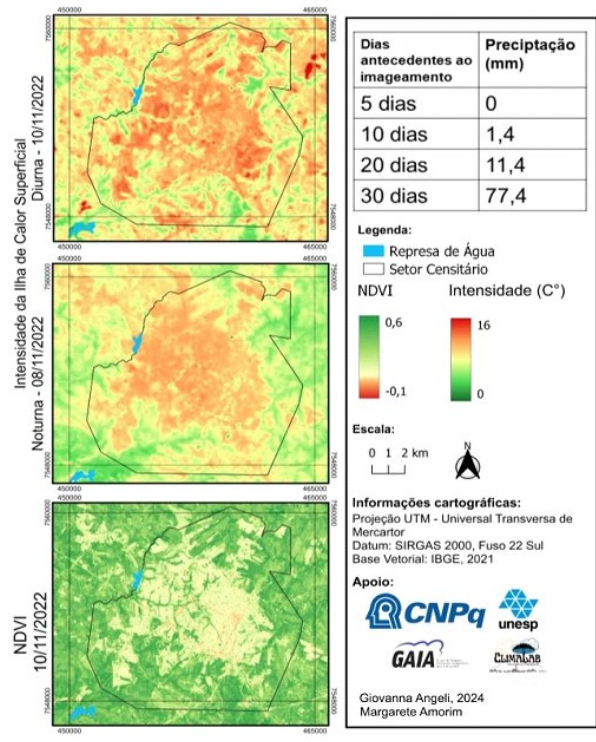
Carta imagem 2 – NDVI e intensidade das ilhas de calor superficiais em novembro de 2022
